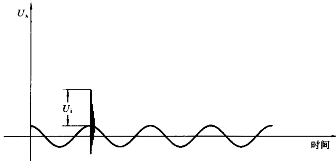
图 8 已叠加随机的非同步高压脉冲的基波交流波形
