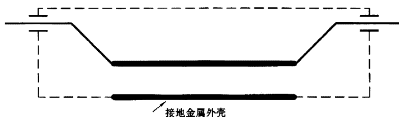
图 4b 非对称使用的穿心电容器(非同轴式)
