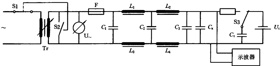
图 7 电容器承受交流电压脉冲典型电路
