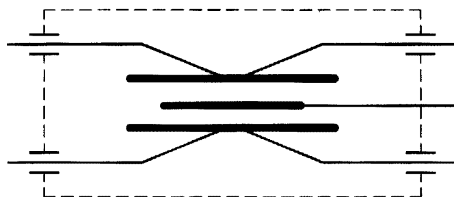
图 4d 多单元穿心电容器
