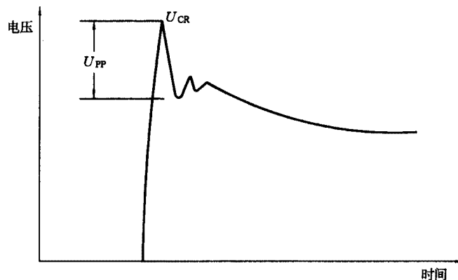
图 6 脉冲波形
