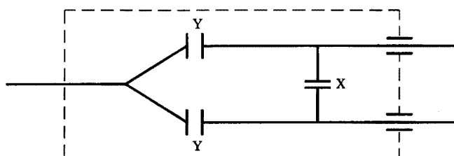
图 5b 三角形连接旁路电容器
