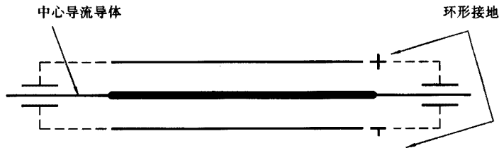
图 3 穿心电容器(同轴式)
